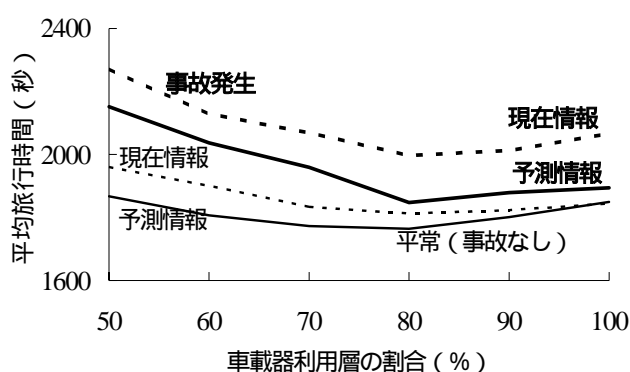
図2 車載器普及率による平均旅行時間の比較
