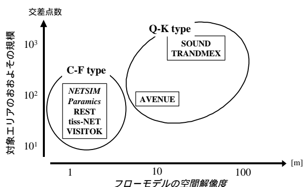
図-2 対象モデルの分類
