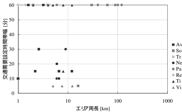
図-10 対象エリア規模と需要設定時間帯幅の関係
